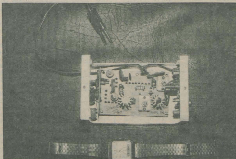
O transmissor é extremamente simples. Para o professor Ubirajara, a vantagem da rádio livre é o seu baixo custo operacional
